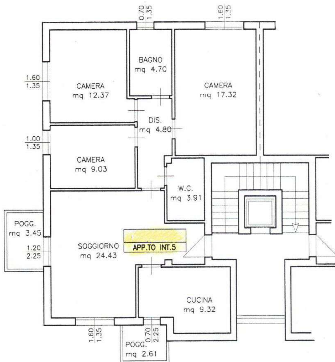
PIANTA PIANO SECONDO H = 2.70
