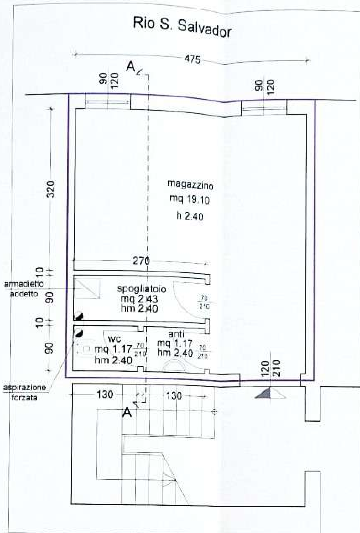
PARTICOLARE PIANO TERRA SCALA 1:50
